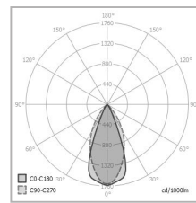
A397IH.F30 Optic Frost 30°
